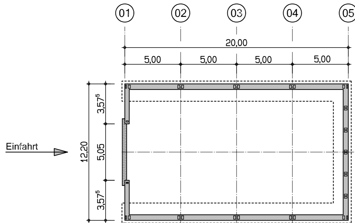
Grundriss Hallenfundament
