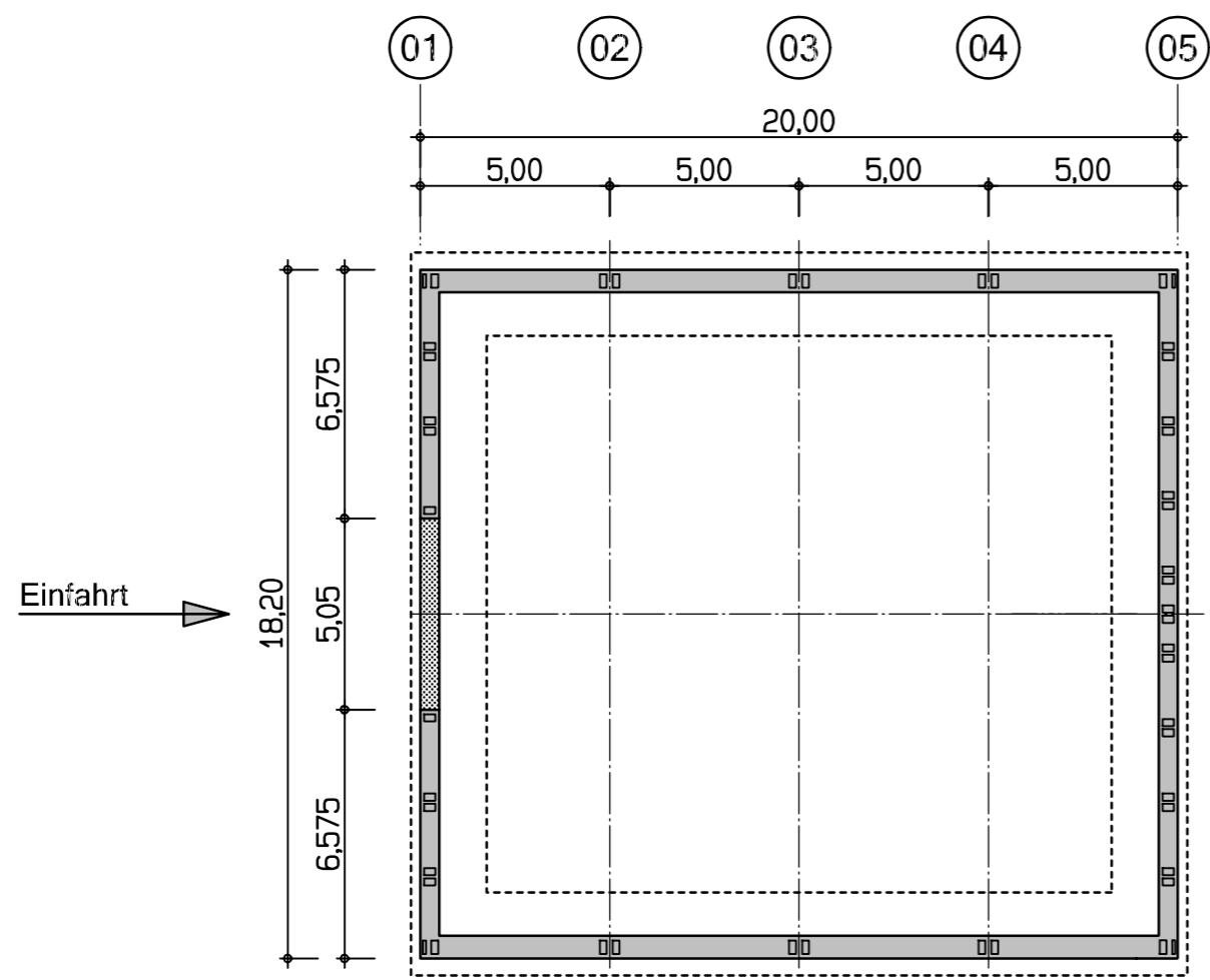
Grundriss Hallenfundament
