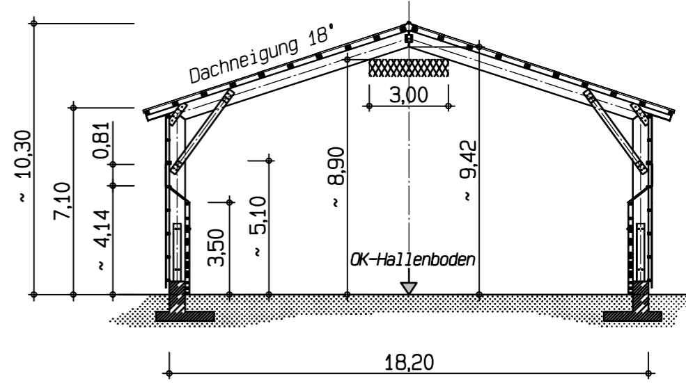
Hallenschnitt
