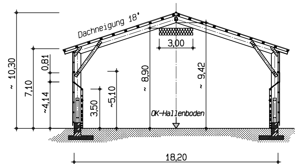
Hallenschnitt
