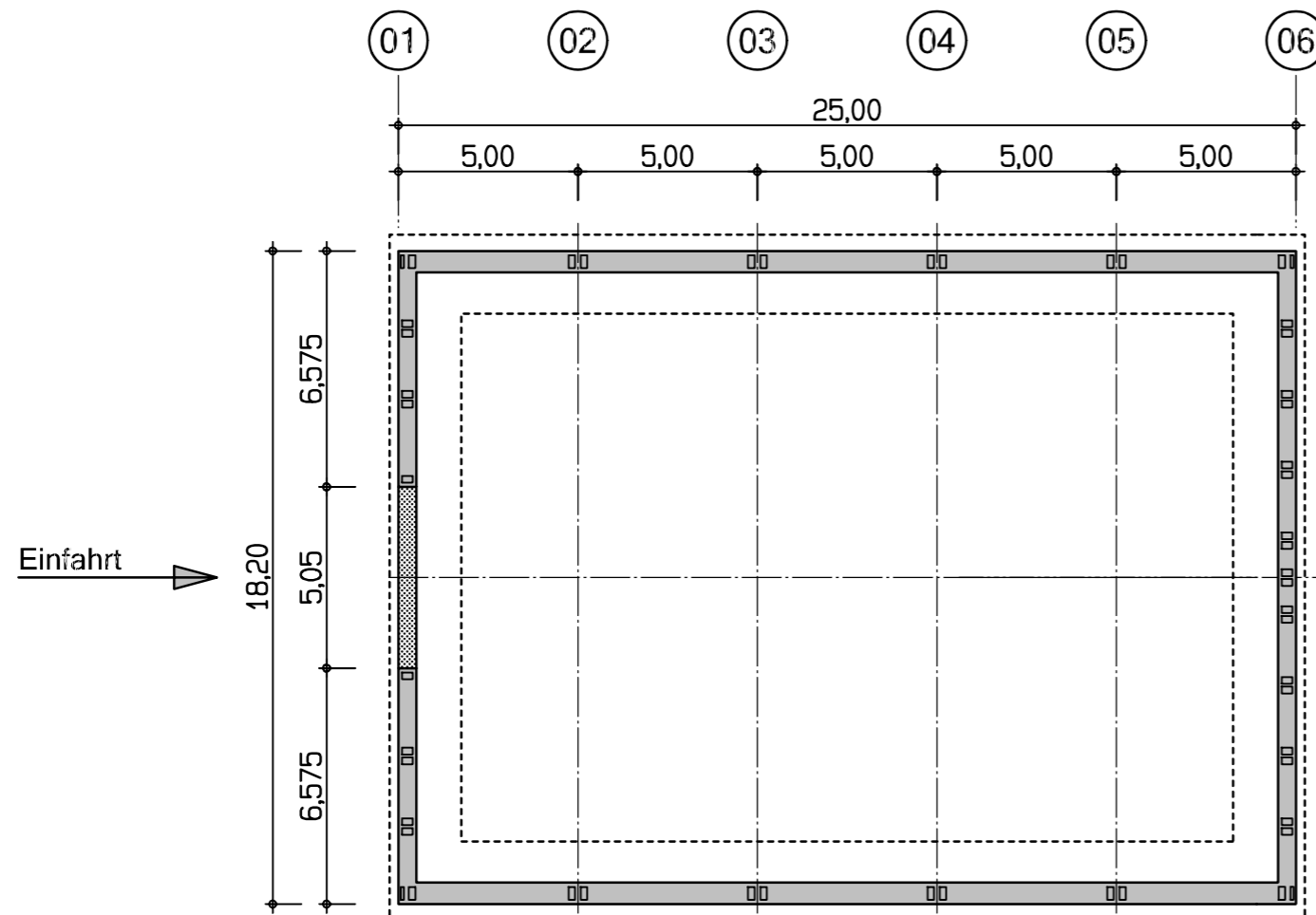
Grundriss Hallenfundament
