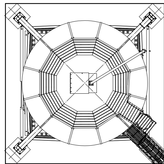
Aufstellfläche footprint
