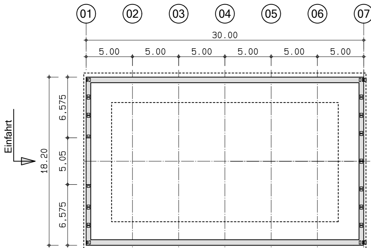
Grundriss Hallenfundament, M1:250
