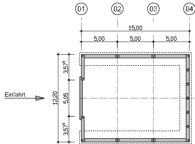
Grundriss Hallenfundament
